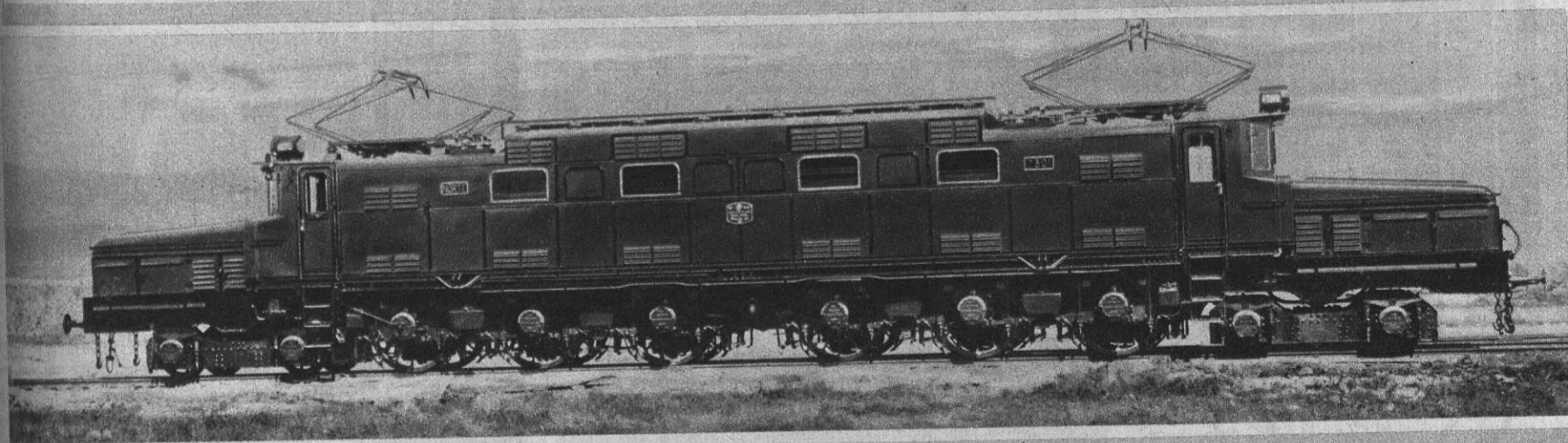
Locomotora eléctrica de gran velocidad, construida en los Talleres Metalúrgicos de Reinosua, en los que se ha logrado nacionalizar su construcción. Tiene una potencia de 4.000 caballos; un peso total de 151 toneladas, y alcanza una velocidad máxima de 110 kilómetros por hora. La Compañía del Norte la tiene en servicio en la línea electrificada de Irún-Alsasua. Esta fotografía demuestra que la industria nacional está lo suficientemente capacitada y preparada para llevar a cabo la electrificación de aquellas líneas ferroviarias que lo requieran por su densidad de circulación y la necesidad de explotarla en las mejores condiciones de economía y rendimiento.
